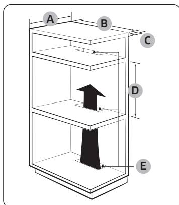
Armário embutido (mm)
