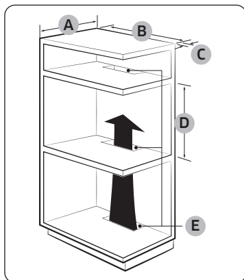
Armario empotrado (mm)
